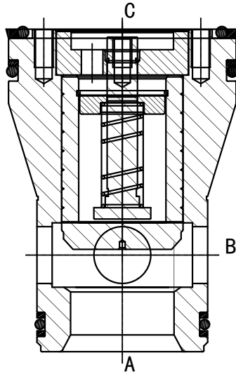
16-63口径 结构图 25-63 diameter Structure Diagram
